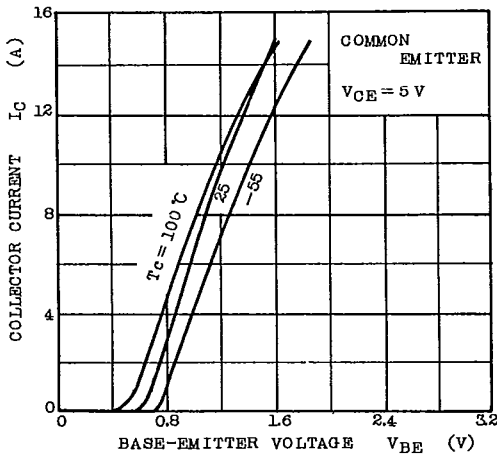
I_C - V_{BE}
